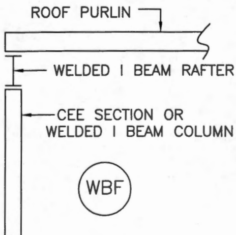
OPTIONAL ENDWALL FRAMING
